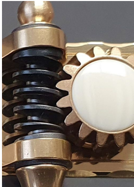
spezial gelagerte Gewindeachse in beiden Böckchen
