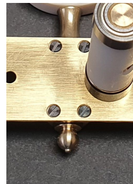
Teile mit Grundplatte verschraubt und nicht vernietet
