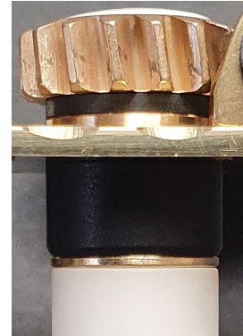
Gleitscheiben aus reibungsarmen Material zwischen Zahnrad und Beinwelle
